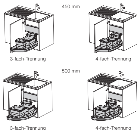
Anordnungsbeispiele
