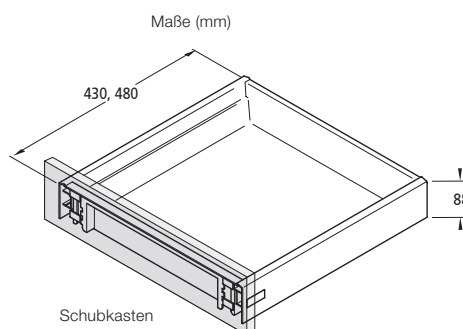
Unterherdschubkasten
